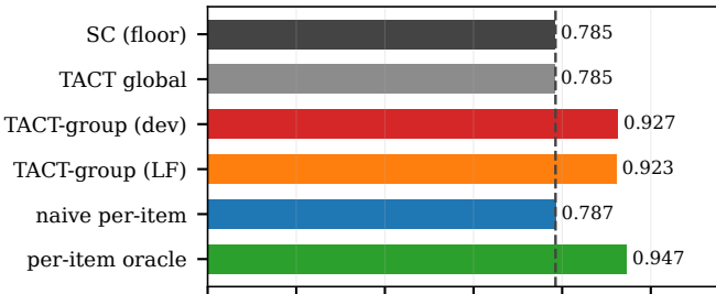
i.i.d.
